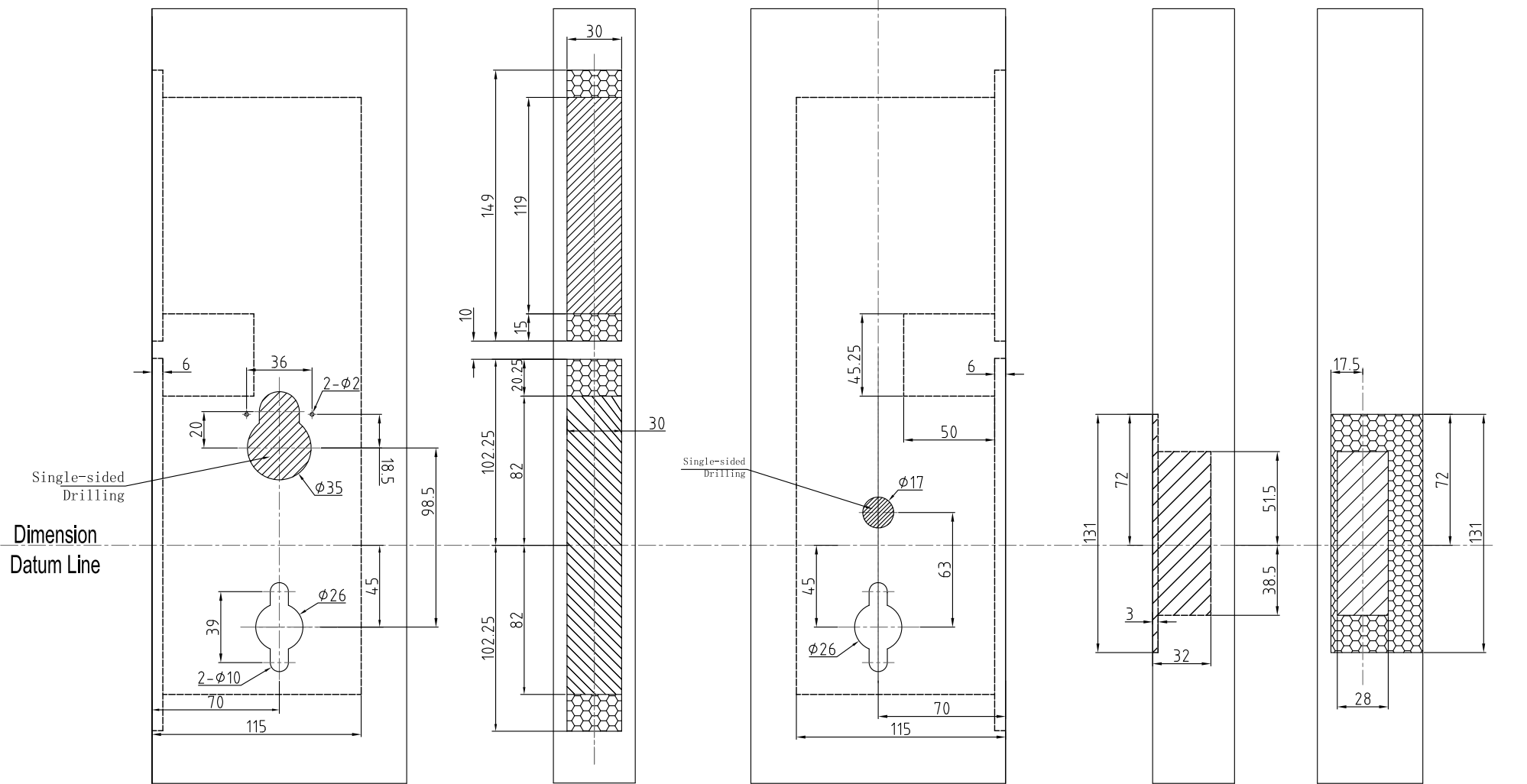
Door Part
